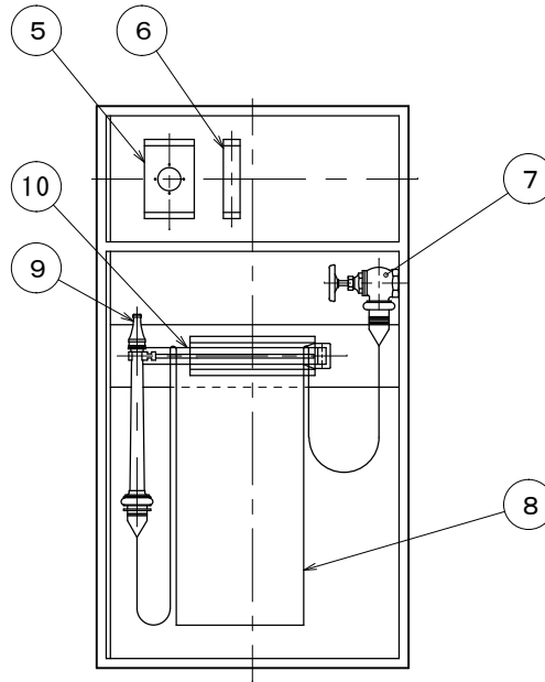
内部配置図
