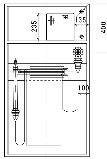
内部配置図
